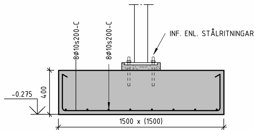
S01 1 : 20 SULA 01
