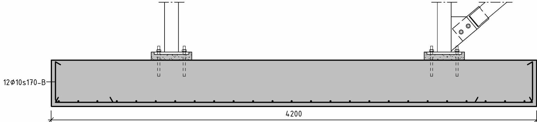
S04b 1 : 20 SULA 04, LÄNGSSEKTION
