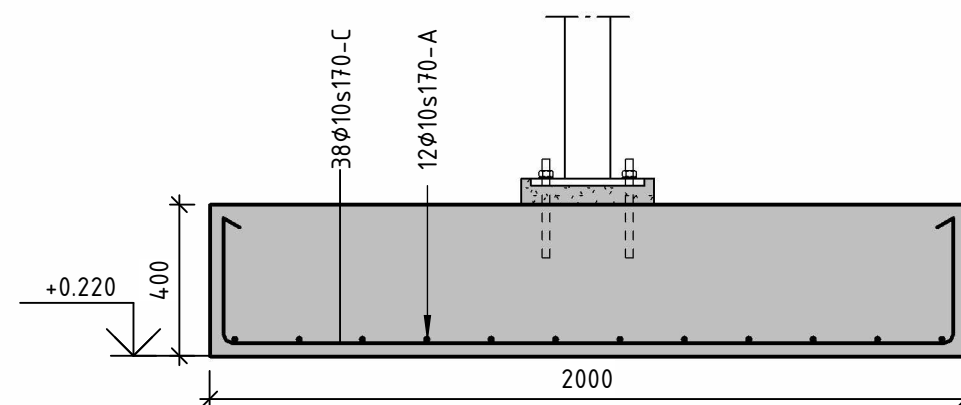
S05a 1 : 20 SULA 05, TVÄRSEKTION
