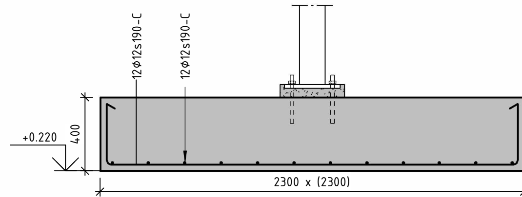
S03 1 : 20 SULA 03
