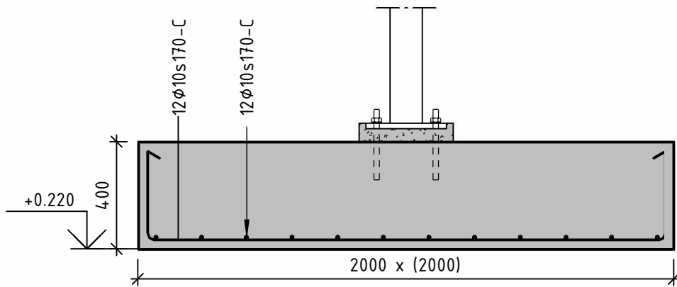
S02 1 : 20 SULA 02
