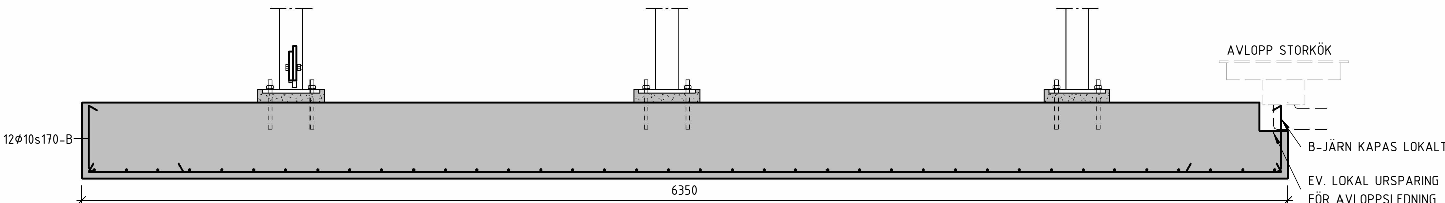
S05b 1 : 20 SULA 05, LÄNGSSEKTION
