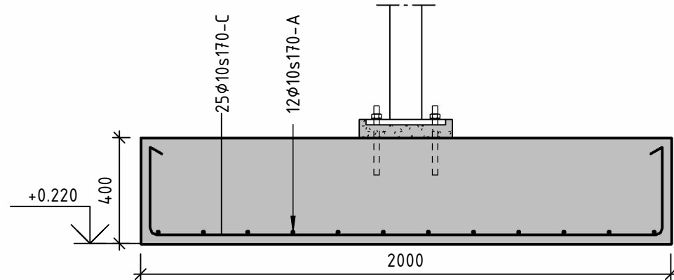
S04a 1 : 20 SULA 04, TVÄRSEKTION
